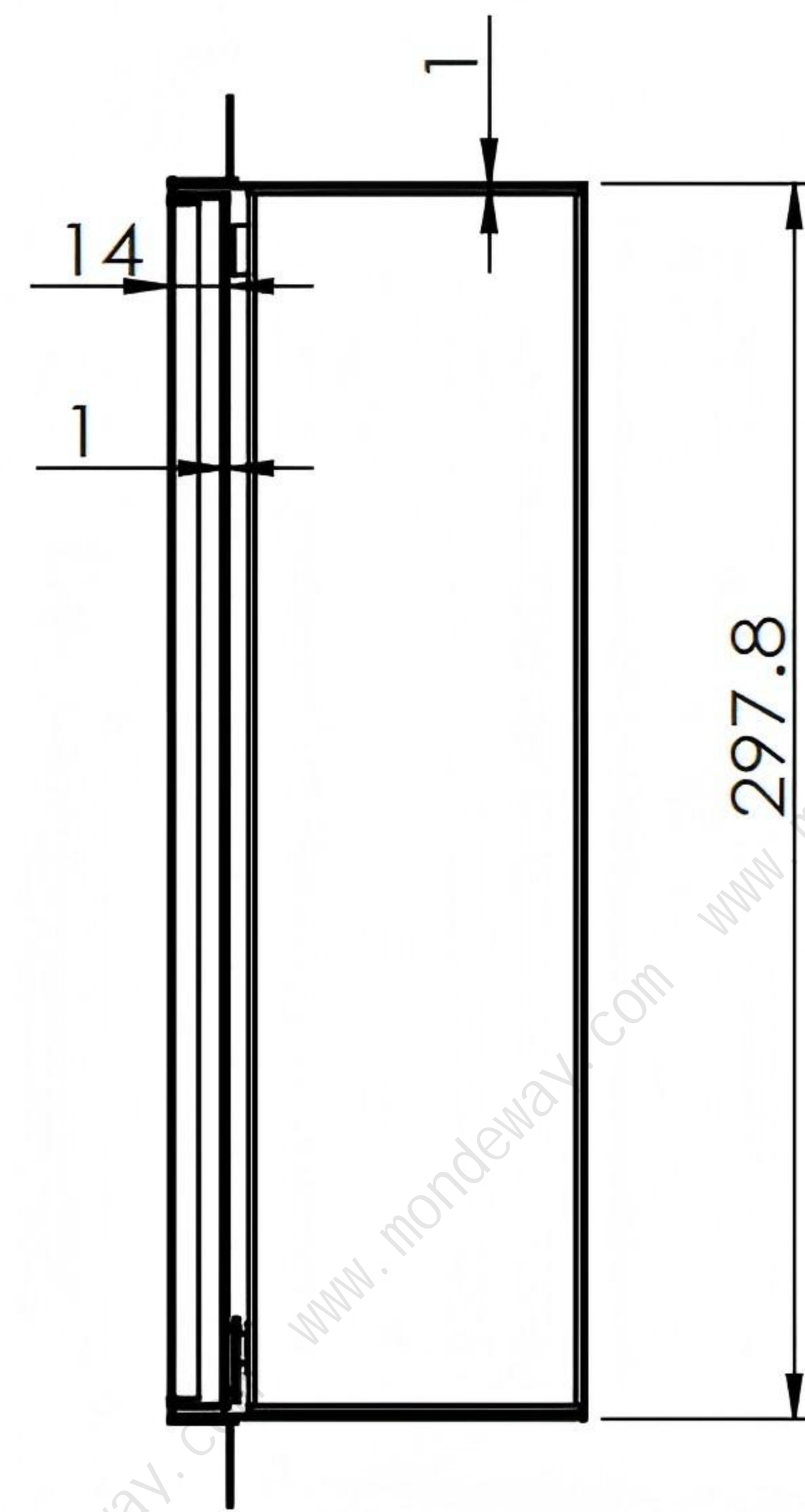
剖面 A-A
