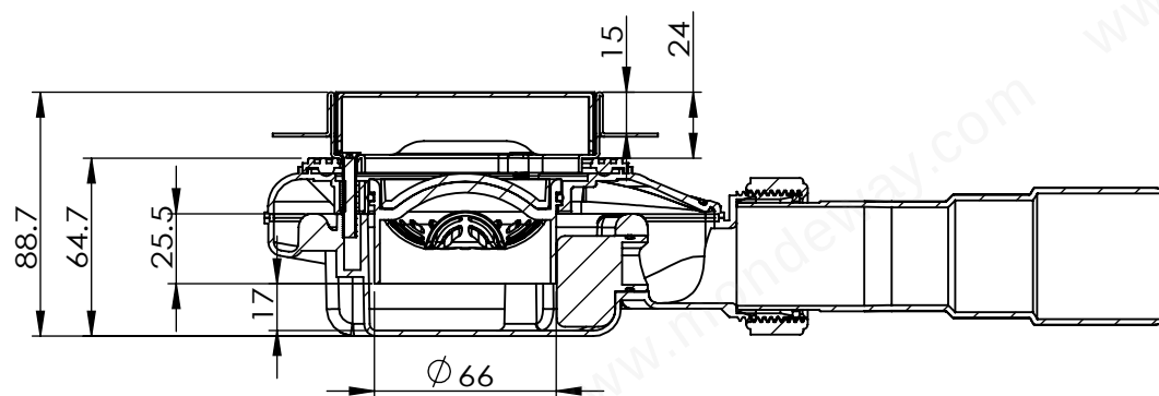
剖面 A-A
