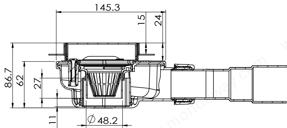
剖面 A-A
